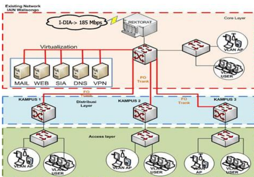
Layout Interkoneksi Infrastruktur Fisik Teknologi Informasi IAIN Walisongo
